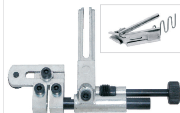
cod. 6764/O3 - parte inferiore portabordatori - lower gauge for binders
