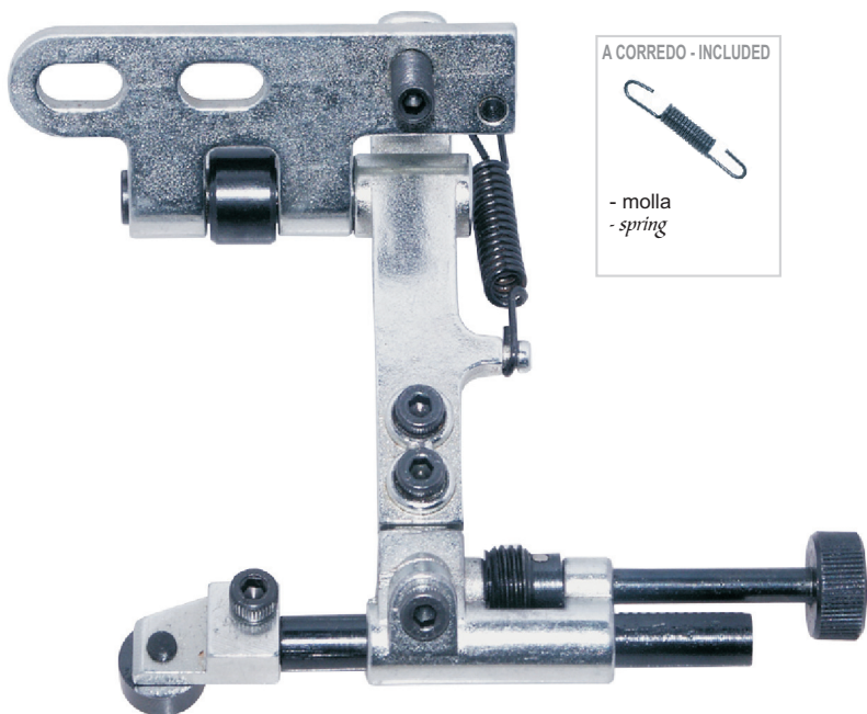
cod. 6764/JE - guida ribaltabile universale - tipo Durkopp - Universal guide - Durkopp type
